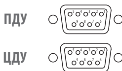
Рис 2 РАЗЪЁМЫ ДИСТАНЦИОННОГО УПРАВЛЕНИЯ ИПГ
