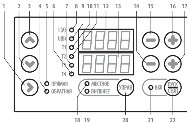
Рис 3 ВНЕШНИЙ ВИД ПАНЕЛИ УПРАВЛЕНИЯ ИСТОЧНИКА ПИТАНИЯ
